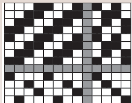
ESQUEMA PARA UN TELAR DE CUATRO PEDALES Y CUATRO PEINES.
