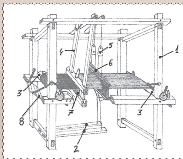
Piezas de un TELAR Nº 1 Armadura Nº 2 Pedales o Esprimideras Nº 3 Usillos o Enjulios Nº 4 Batán Nº 5 Poleas Nº 6 Peines Nº 7 Puga Nº 8 Apoyo.
