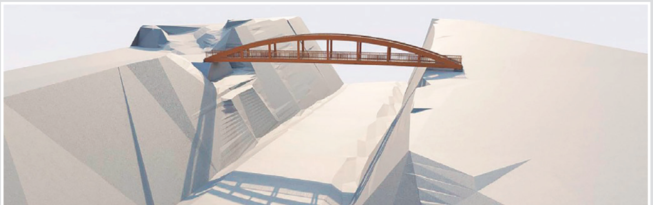
PROYECTO DEL PUENTE DE MADERA DE 41 M. SOBRE LA N-240
